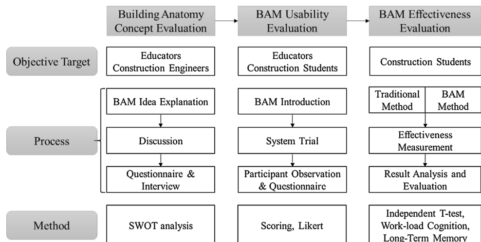
Fig. 11 Evaluation framework
